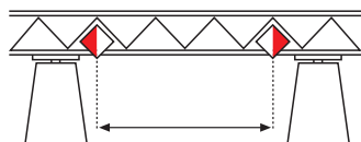
Durchfahrverbot außerhalb des von den Tafeln begrenzten Raumes (gilt auf Seeschiffahrtsstraßen nicht für kleine Fahrzeuge)
